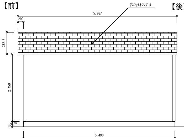
【右面図】
