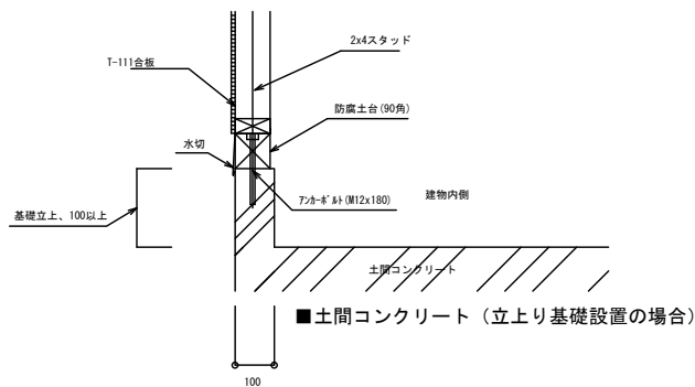
【正面】
