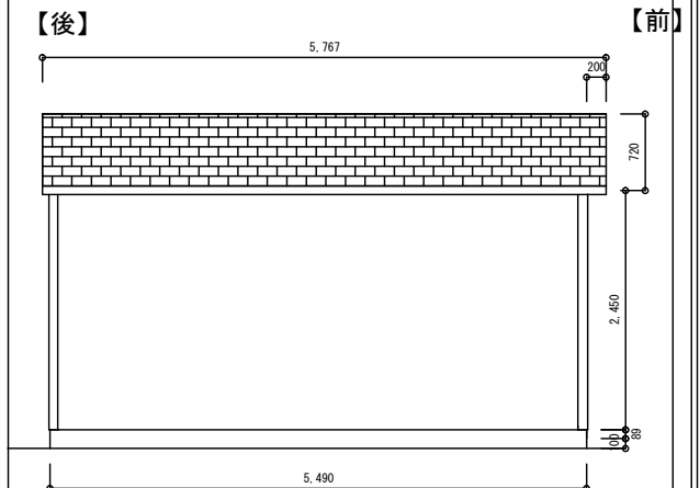
【左面図】
